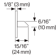
Striker
