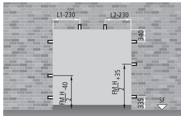
Ouverture gauche SX
