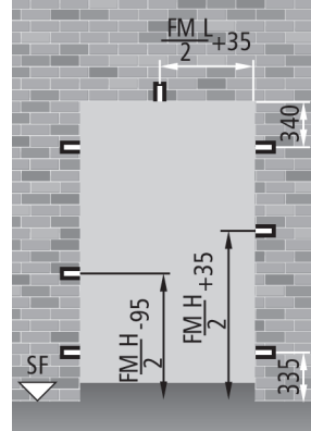
Porte à un vantail Ouverture droite DX
