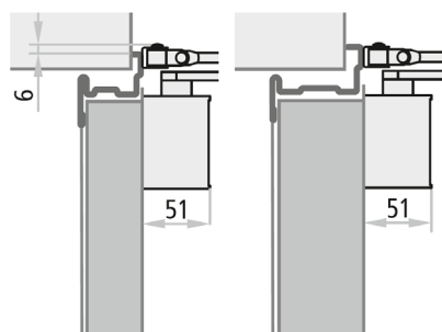
CP1 REVER CP1 UNIVER (côté tirant)
