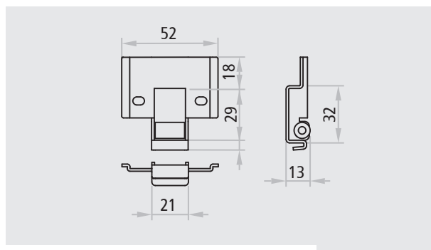
Gâche haute vantail passif PROGET et autres multiusage
