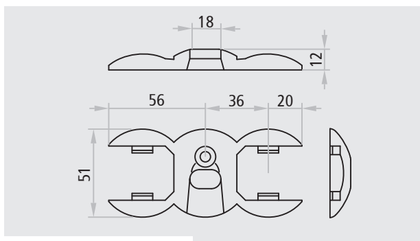
Gâche de sol vantail passif REVER
