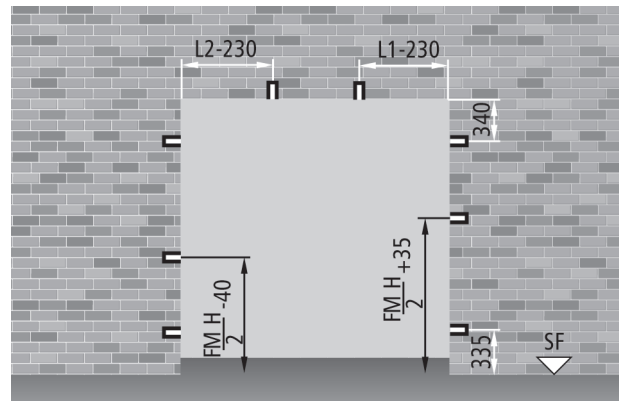
Porte à deux vantaux Ouverture droite DX
