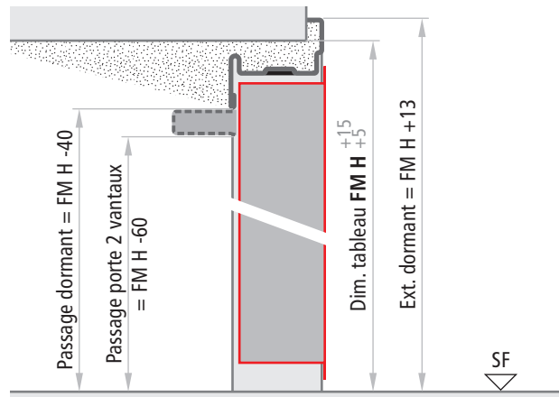
Porte sans battue inférieure - Coupe verticale
