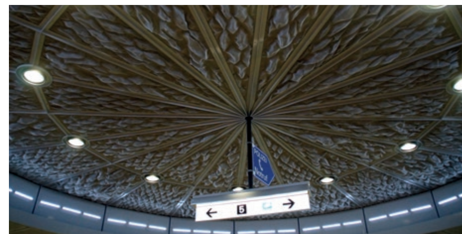
Tela de acero inoxidable deformado en forma tridimensional para el mejoramiento de la acústica ambiental. Ferrocarril ligero, Colonia, Alemania, MONTANA.
