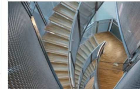
La tela de acero inoxidable como relleno elegante de barandas. St. Michael's Hospital, Toronto, Canadá.
