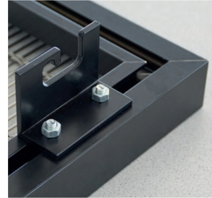
Posibilidades de suspensión para elementos de armazón.
