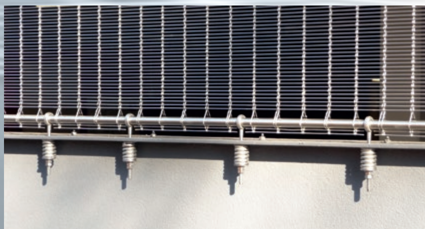
Fijación inferior: varilla redonda con tornillo de ojo y resorte de compresión.
