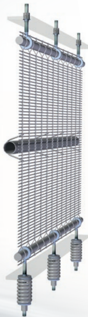
Tecnología de fijación para fachadas de tela de cable.
