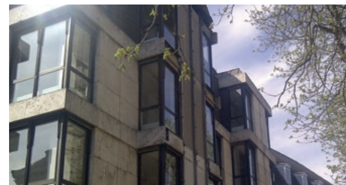
Lo antiguo se convierte en nuevo. El revestimiento de la fachada con tela para la arquitectura de HAVER DOKAWELL-MONO 3601 en el Palacio de Congresos, Baden-Baden, Alemania.
