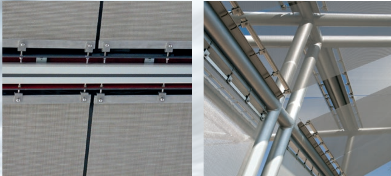
Sistemas de fijación no desmontables para techos con pliegue tensor y tornillo de horquilla.
