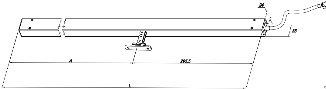
Actuators dimensions
