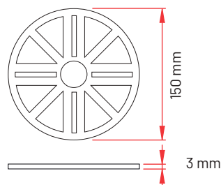
LH 3 - Livellatore in gomma LH3 LH 3 - Rubber shim
