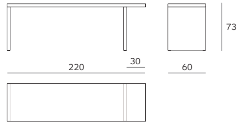
Mod. 0661-01
