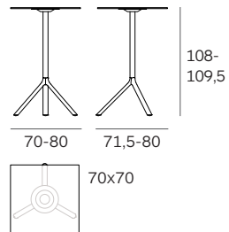
Mod. 9580-71 (70x70)
