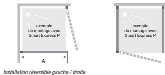
Installation réversible gauche / droite
