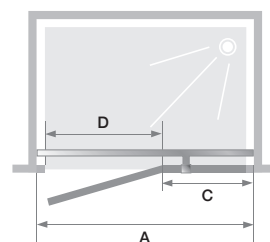
Charnières à droite
