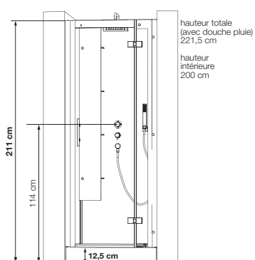
Cotes pour le modèle C90 niche
