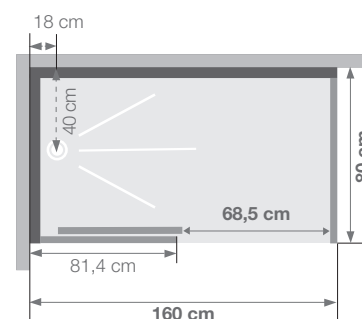
Installation réversible gauche / droite
