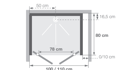
Kineprime 100 x 80 niche - version mécanique - 2 portes pivotantes
