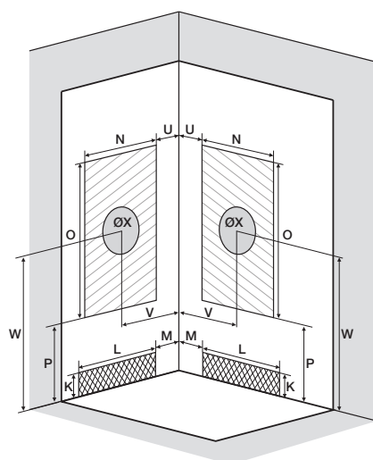
Cotes pour le modèle C80 niche
