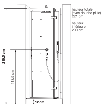
Cotes pour le modèle C80 niche
