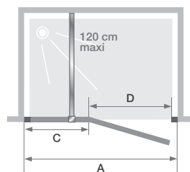
Tailles \geq 110 cm Installation réversible gauche / droite
