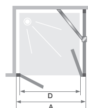
Montage en angle avec Smart Express+ Fixe
