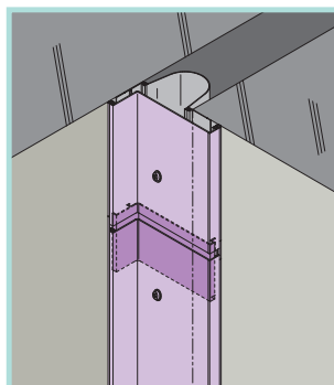
8 外壁コーナー（直線） 外壁コーナー
