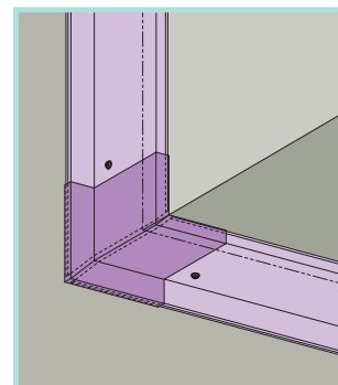
9 外壁コーナー（出隅） 外壁コーナー
