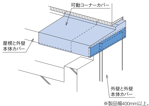
可動タイプ [ 屋根と外壁：外壁と外壁 ]
