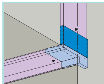
6 外壁と外壁 天井と外壁（出隅）
