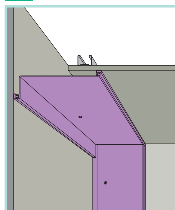
3 天井と内壁（入隅） 内壁コーナー（入隅）
