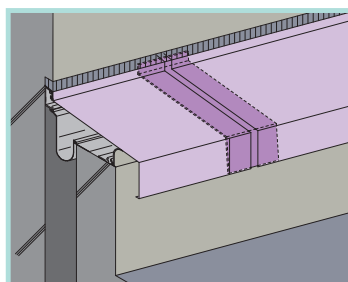
17 屋根と外壁（直線） 屋根と外壁
