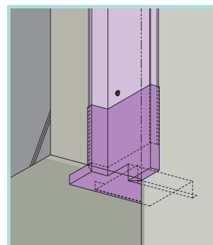
15 外壁コーナー（反転） 外壁コーナー
