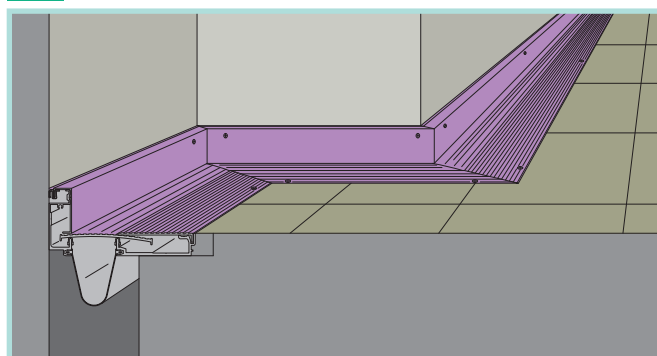
5 床と内壁（平面コーナー） 床と内壁
