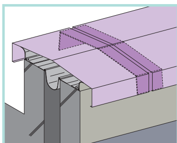
16 屋根と屋根（直線） 屋根と屋根
