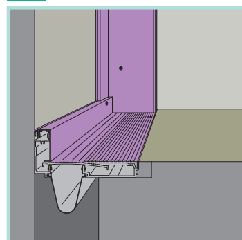
6 床と内壁（入隅） 内壁コーナー（入隅）
