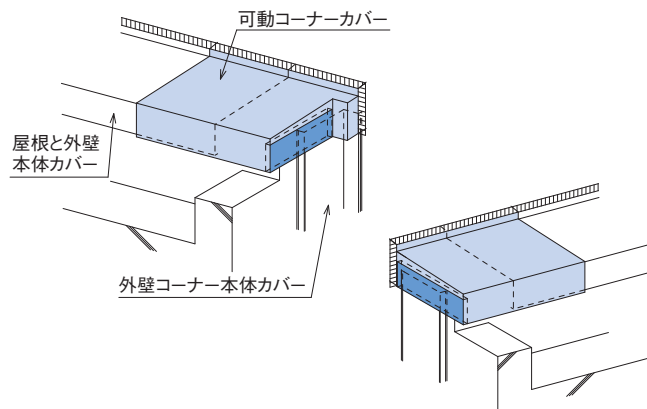
可動タイプ [ 屋根と外壁：外壁コーナー ]
