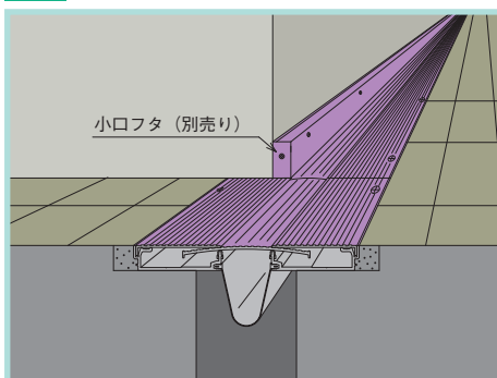
5 床と床（直線） 内壁コーナー（直線）
