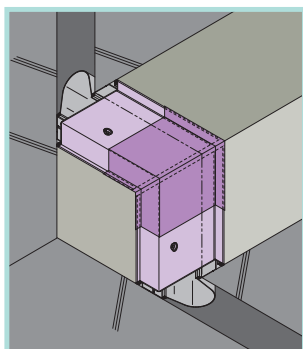
10 外壁コーナー（入隅） 外壁コーナー
