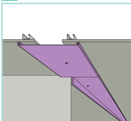
2 天井と天井（直線） 内壁コーナー（直線）
