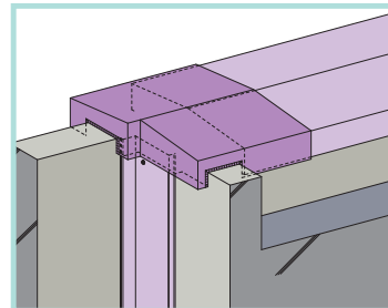
6 屋根と屋根 外壁コーナー（出隅）
