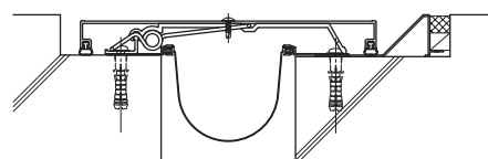
Y方向可動時
