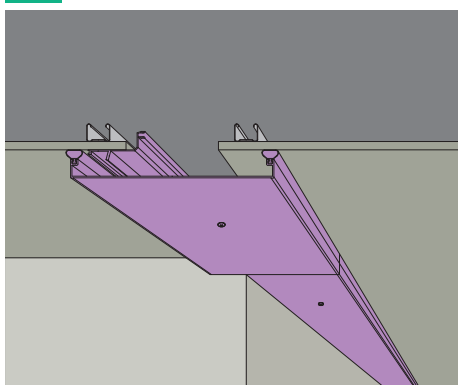
2 天井と天井 内壁コーナー（直線）
