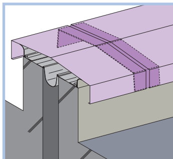
16 屋根と屋根（直線） 屋根と屋根
