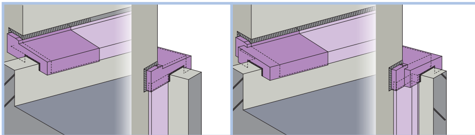
4 屋根と外壁（反転） 外壁コーナー
