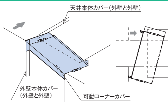
Y方向可動時
