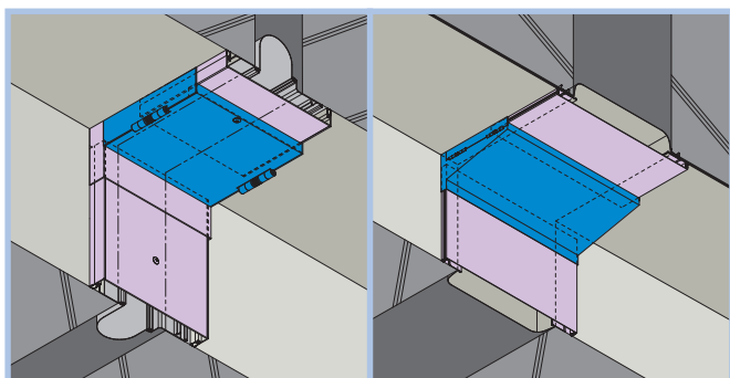
9 外壁と外壁（入隅） 天井と天井
