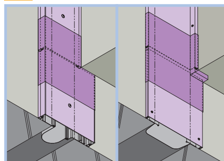
14 外壁コーナー 外壁と外壁（直線）
