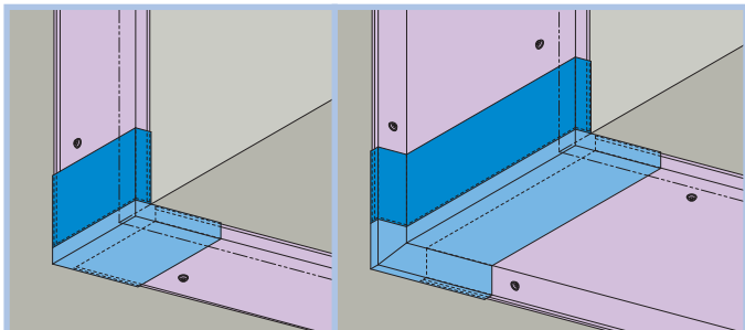
7 外壁コーナー (出隅) 天井と外壁
