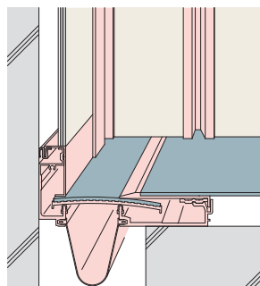
床と内壁・内壁コーナー
