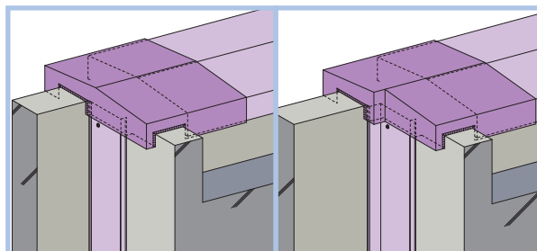
6 屋根と屋根（出隅） 外壁コーナー
