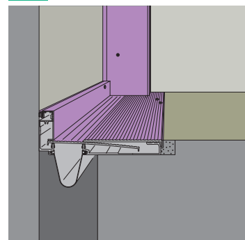
6 床と内壁 内壁コーナー（入隅）
