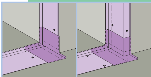
7 外壁コーナー 外壁と外壁（出隅）
