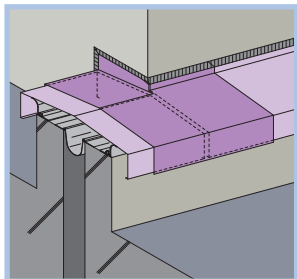
3 屋根と屋根（出隅） 屋根と外壁
