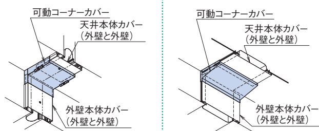
天井と天井：外壁と外壁
