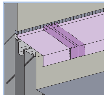
17 屋根と外壁（直線） 屋根と外壁
