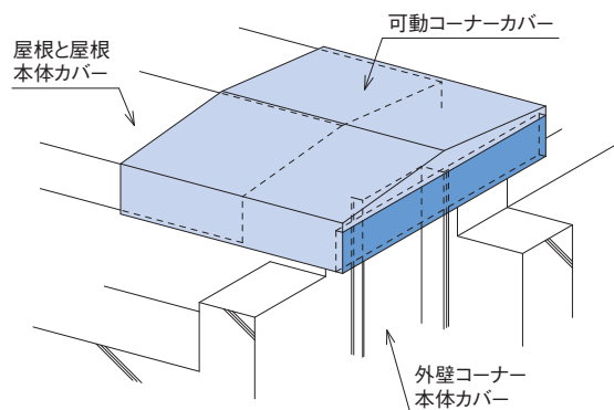
可動タイプ [ 屋根と屋根：外壁コーナー ]
