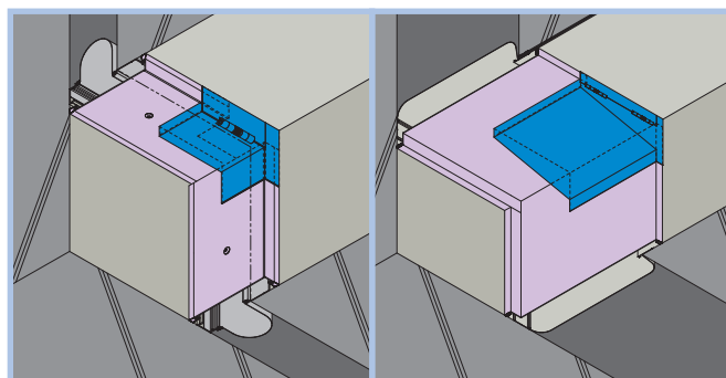
10 外壁コーナー（入隅） 天井と外壁
