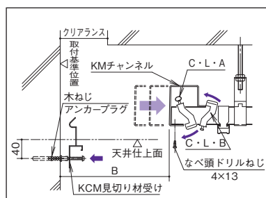
KCM見切り材受け 切欠き詳細
