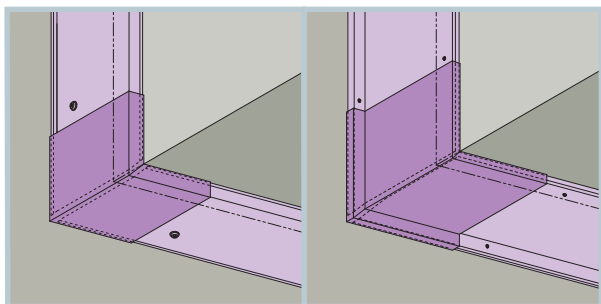
9 外壁コーナー（出隅） 外壁コーナー
