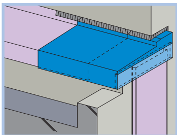
3 屋根と外壁 (出隅) 外壁と外壁
