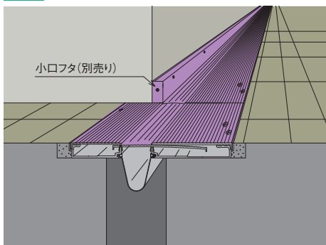
5 床と床 内壁コーナー（直線）
