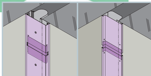
8 外壁コーナー 外壁コーナー（直線）
