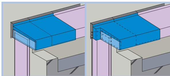
4 屋根と外壁 (出隅) 外壁コーナー
