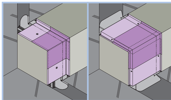
10 外壁コーナー（入隅） 外壁コーナー
