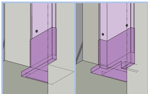
15 外壁コーナー（反転） 外壁コーナー
