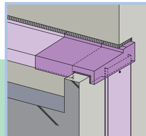
2 屋根と外壁 外壁と外壁（出隅）
