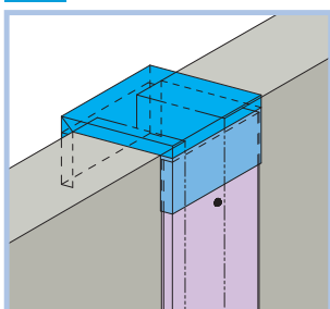
11 手摺壁天端取合い
