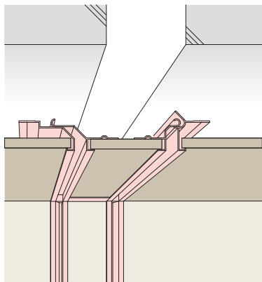
天井と天井・内壁と内壁
