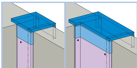
12 手摺壁天端取合い
