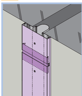
11 外壁と外壁 外壁と外壁（直線）
