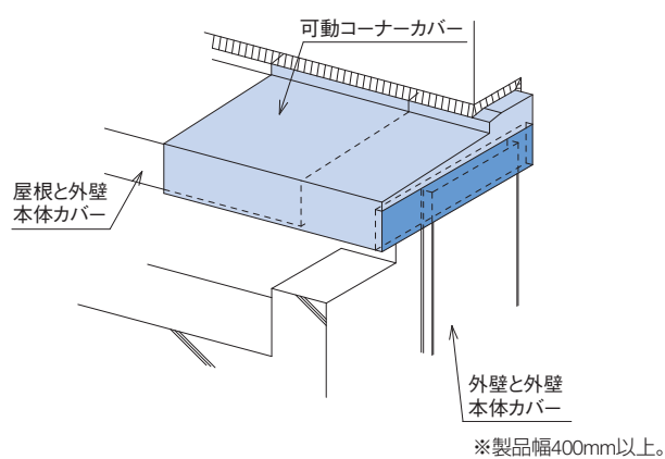
可動タイプ [ 屋根と外壁：外壁と外壁 ]
