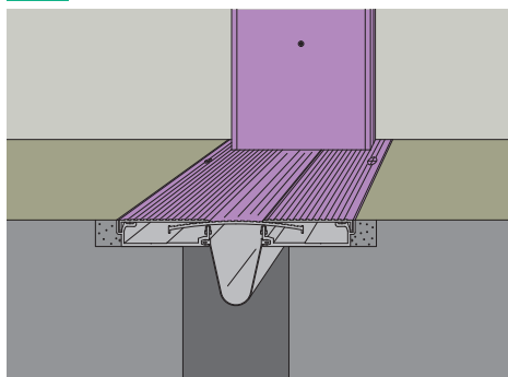
4 床と床 内壁と内壁（入隅）
