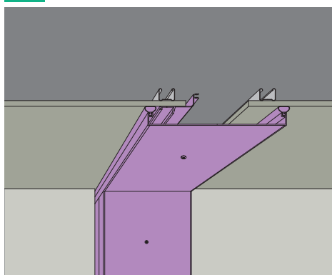
1 天井と天井 内壁と内壁（入隅）
