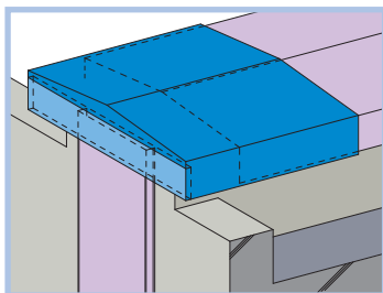
1 屋根と屋根（出隅） 外壁と外壁
