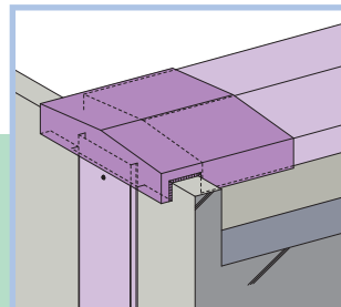
1 屋根と屋根 外壁と外壁（出隅）
