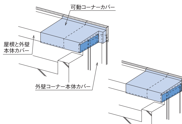
可動タイプ [ 屋根と外壁：外壁コーナー ]
