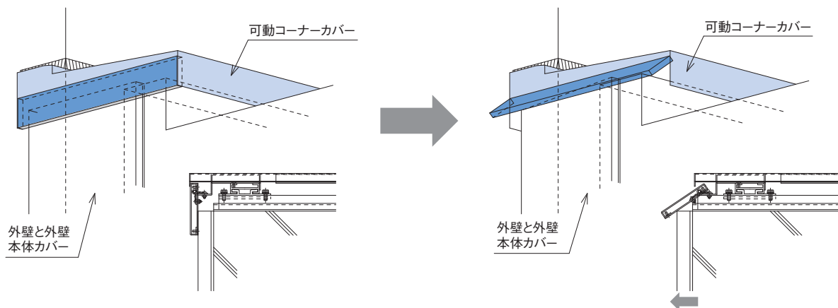
可動状態図
