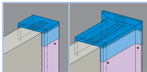
13 手摺壁天端取合い
