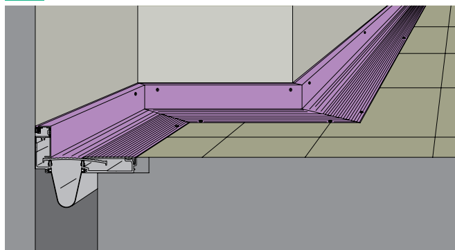
8 床と内壁 床と内壁（平面コーナー）
