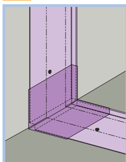
12 外壁と外壁 外壁と外壁（出隅）
