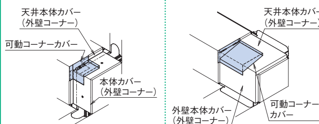
天井と外壁：外壁コーナー (左)
