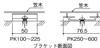
ブラケット断面図
