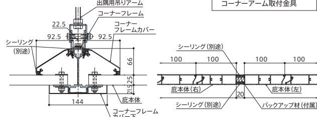
d-d' 断面図 (コーナーフレーム)
