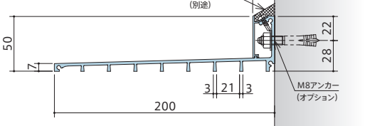
EV-200R 200mm (リップタイプ)
