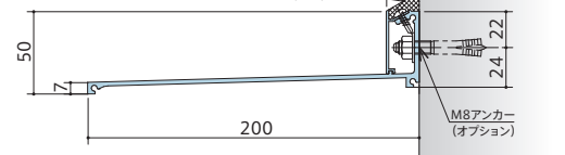
EV-200F 200mm (フラットタイプ)
