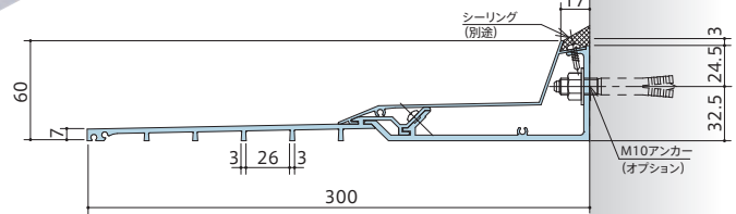
EV-300R 300mm (リップタイプ)
