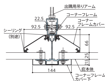
d-d'断面図(コーナーフレーム)
