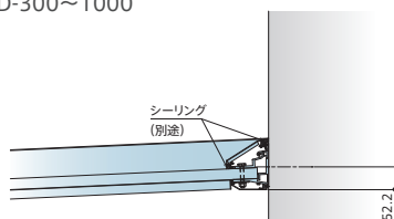
a-a' 断面図(コーナ一部)
