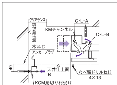
KCM見切り材受け 切欠き詳細
