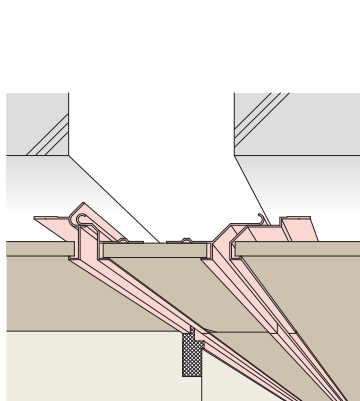
天井と天井・天井と内壁
