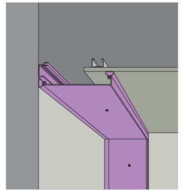
3 天井と内壁 外壁と外壁（出隅）
