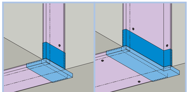
8 外壁コーナー (出隅) 天井と天井
