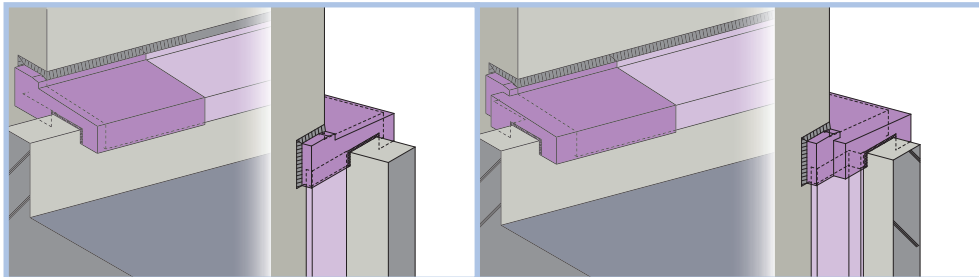
4 屋根と外壁（反転） 外壁コーナー
