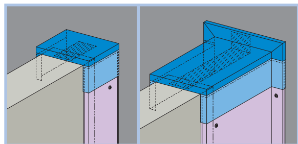
13 手摺壁天端取合い
