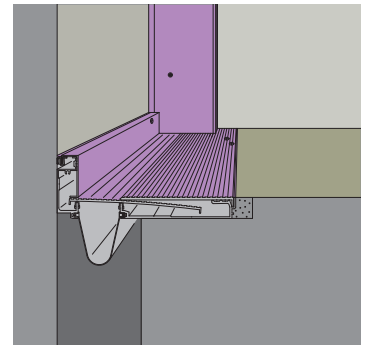
6 床と内壁 内壁コーナー（入隅）
