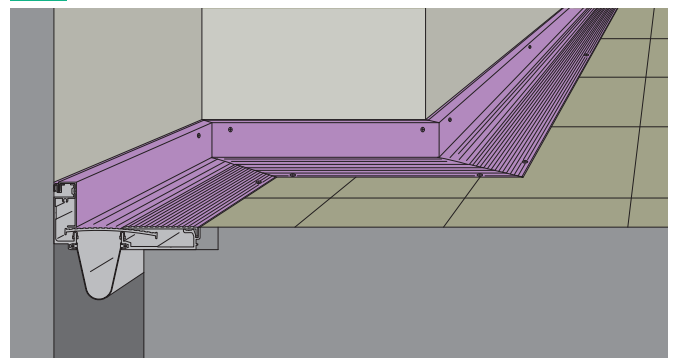
8 床と内壁 床と内壁（平面コーナー）
