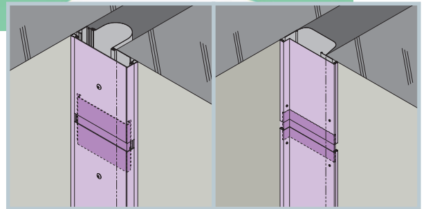
8 外壁コーナー 外壁コーナー (直線)
