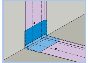
5 外壁と外壁 (出隅) 天井と天井
