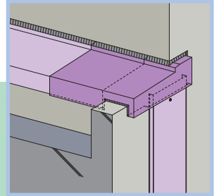
2 屋根と外壁 外壁と外壁 (出隅)
