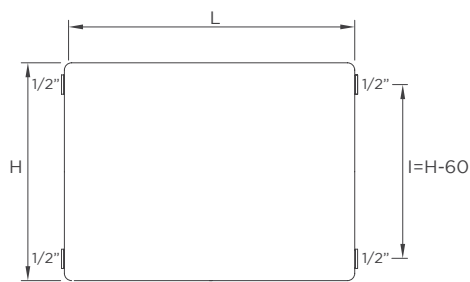
Vista frontale
