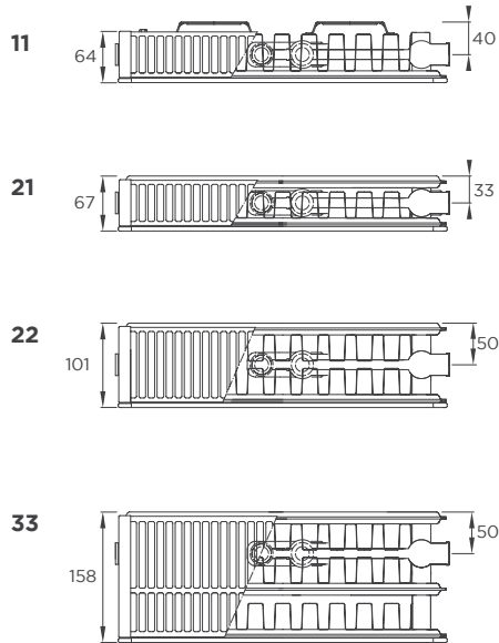
Vista superiore
