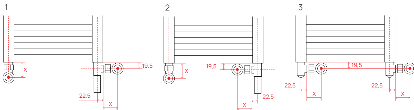
A Valvola (entrata) B Detentore (uscita) C Raccordo a "T"
