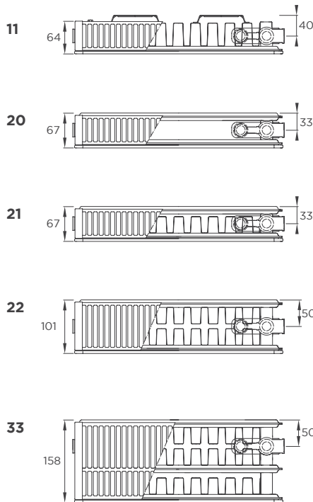
Vista superiore
