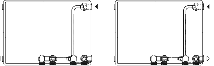
Connessioni possibili
