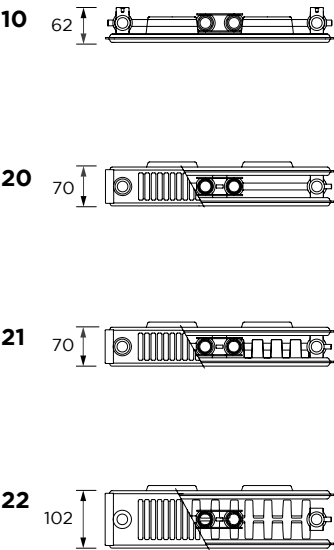
Vista superiore
