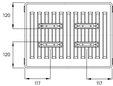
Vista superiore
