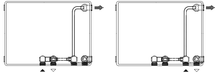
Connessioni possibili
