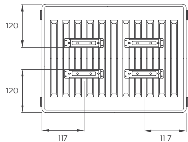
Vista superiore
