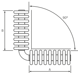
Attacco laterale
