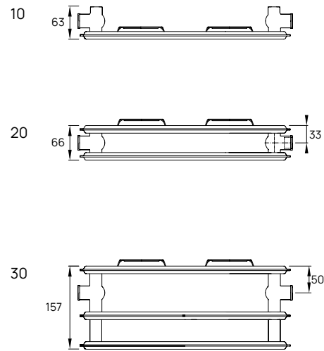
Vista superiore
