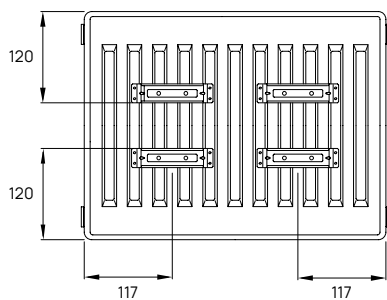
Vista superiore
