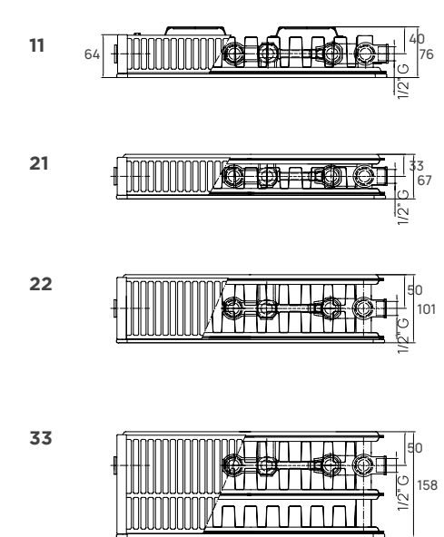
Vista superiore
