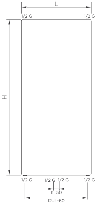
Vista frontale
