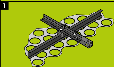
Rostwinkel, Fix-Clip und C-Profil L-shaped primary carrier, fix-clip and C-profile Porteur primaire L, clip de fixation et Porteur-C
