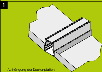
Aufhängung der Deckenplatten Moving the ceiling panel Déplacement coulissant du panneau
