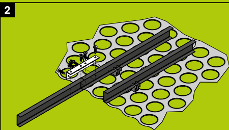
C-Profil mit Adapter für die Montage des Deckenelements C-profile with adapter piece for ceiling element assembly Profil en C avec adaptateur pour le montage des éléments de plafond
