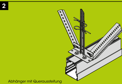
Abhänger mit Queraussteifung Hanger with lateral bracing Suspension avec renforcement transversal
