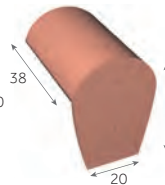
Faîtière d'about conique de 40 (fin)
