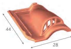
Tuile châtière (ouverture de 21 cm²) 3,8 kg/pièce
