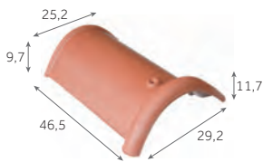
Faitière/arêteur demi-ronde de 40
