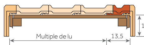
Montage avec rives à rabat et demi-tuiles
