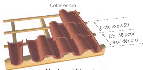
Montage à l'égout avec Canal Sablière et Demi-Tuile
