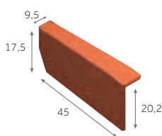
Rive à rabat gauche 2,7 à 3,3 au m 3,7 kg/pièce
