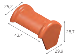
Faîtière d'about demi-ronde (fin) 5,8 kg/pièce
