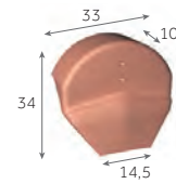
Fronton de rive ronde de 50 (grand modèle)
