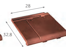
Tuile et demie d'about
