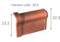
Rive universelle de 33 droite 3 au m 3,4 kg/pièce
