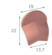
Écusson de rive ronde conique de 40
