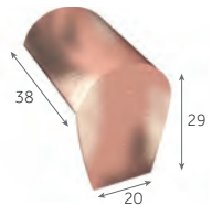
Faitière d'about conique de 40 (fin) 5,1 kg/pièce
