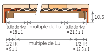
Montage avec tuiles de rives
