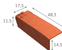
Demi-tuile de rive gauche 1,4 à 1,7 au m 3,6 kg/pièce
