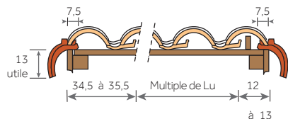
Montage avec rive ronde et demi-tuile
