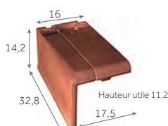
Demi-tuile de rive gauche
