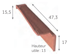
Rive à rabat droite
