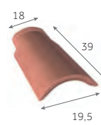
Canal couvert 3/4 de pureau 4 au m 2 kg/pièce
