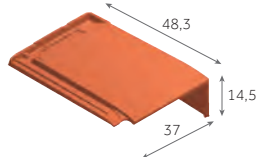
Tuile de rive droite 1,4 à 1,7 au m 6,2 kg/pièce
