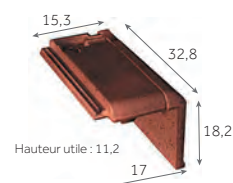
Demi-tuile de rive droite
