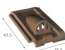
Tuile chatière grillagée (ouverture 12 cm²) 3,5 kg/pièce
