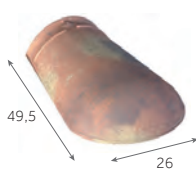
Arêtier d'about conique de 50 4 kg/pièce
