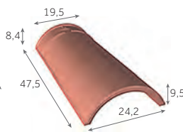
Faîtière/arêtier conique de 40 (selon coloris)
