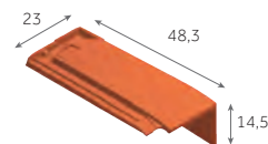
Demi-tuile de rive droite 1,4 à 1,7 au m 3,9 kg/pièce
