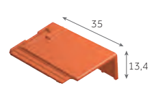
Tuile de rive droite 2 au m 4,6 kg/pièce
