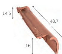
Rive ronde droite 2,5 au m 3,5 kg/pièce
