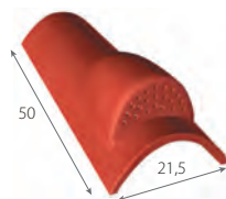
Tuile chatière grillagée (ouverture de 16 cm²) 3,1 kg/pièce
