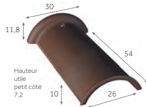
Faîtière demi-ronde de 50
