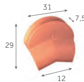
Fronton de rive ronde 3 kg/pièce
