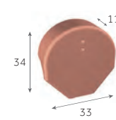
Fronton de rive à rabat de 50 (grand modèle)
