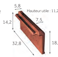
Rive à rabat droite
