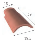
Canal sablière 3,5 au m 2,6 kg/pièce
