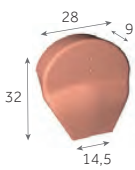
Fronton de rive ronde de 40 (petit modèle)
