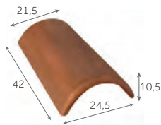
Faitière/arêtier de 42 à recouvrement
