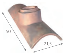
Tuile à douille (Ø intérieur du tuyau d'évacuation : 100 mm) 3,4 kg/pièce
