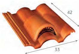
Tuile chatière grillagée (ouverture 18 cm 2 )
