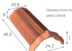
Arêtier à emboîtement de 40 2,5 au m 3,5 kg/pièce
