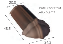
Arêtier d'about à emboîtement de 40
