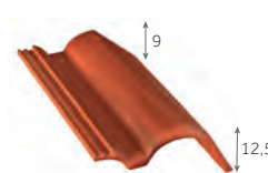
Tuile de rive ronde raccord droite 4,4 kg/pièce
