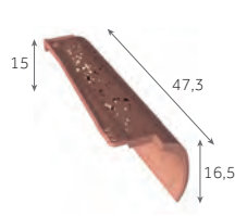
Rive ronde droite 2,7 au m 2,8 kg/pièce
