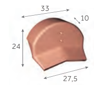
Fronton de rive bardelis de 50 (grand modèle)
