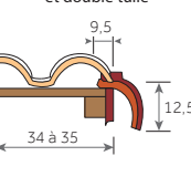
Montage avec rive ronde et double tuile
