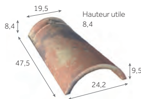
Faîtière/arêteur conique de 40 2,5 au m 3 kg/pièce
