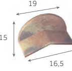
Écusson de rive bardelis demi-ronde de 50 0,8 kg/pièce
