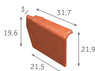
Rive à rabat gauche 4,1 au m 2,5 kg/pièce
