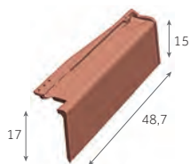
Rive à rabat droite 2,5 au m 3,3 kg/pièce
