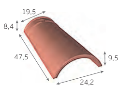
Faitière/arêteur conique de 40
