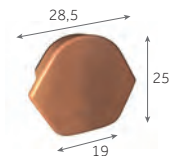
Fronton pour Faitière/arêtier de 42 à recouvrement
