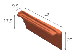
Rive à rabat droite 2,7 à 3,3 au m 3,7 kg/pièce
