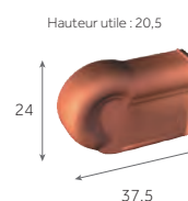
About de rive de 33 droite 3,2 kg/pièce
