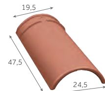
Faîtière/arêtier conique de 40 2,5 au m 3,3 kg/pièce
