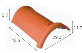
Faîtière/arêtier demi-ronde de 40 ventilée 2,5 au m 4 kg/pièce
