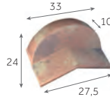
Fronton de rive bardelis de 50 (grand modèle) 2,5 kg/pièce
