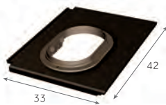
DUROVENT Tuile à douille INNOTECH® (Ø 110 à 160 mm) 4 kg/pièce
