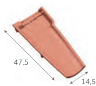
Canal sablière 3,5 au m 2,6 kg/pièce
