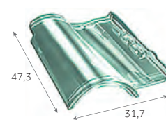
Tuile en verre GALLEANE®10 6,3 kg/pièce
