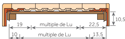
Montage avec rives à rabat
