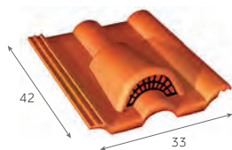
Tuile chatière grillagée (ouverture 18 cm 2 ) 5,7 kg/pièce
