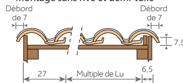
Montage sans rive et demi-tuile
