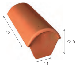
Faîtière d'about de 42 (début)
