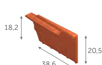
Rive à rabat droite 4 au m 2,9 kg/pièce
