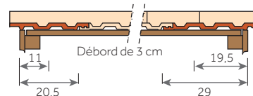
Montage avec tuiles d'about
