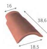
Canal couvert 3/4 de pureau
