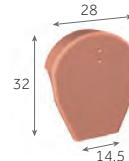
Fronton de rive à rabat (petit modèle)
