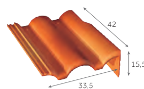
Tuile de rive universelle droite 3,2 au m 7,1 kg/pièce
