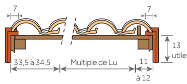
Montage avec rive à rabat et demi-tuile
