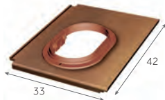
DUROVENT Tuile à douille NOBILÉE® universelle (Ø 110 à 160 mm)
