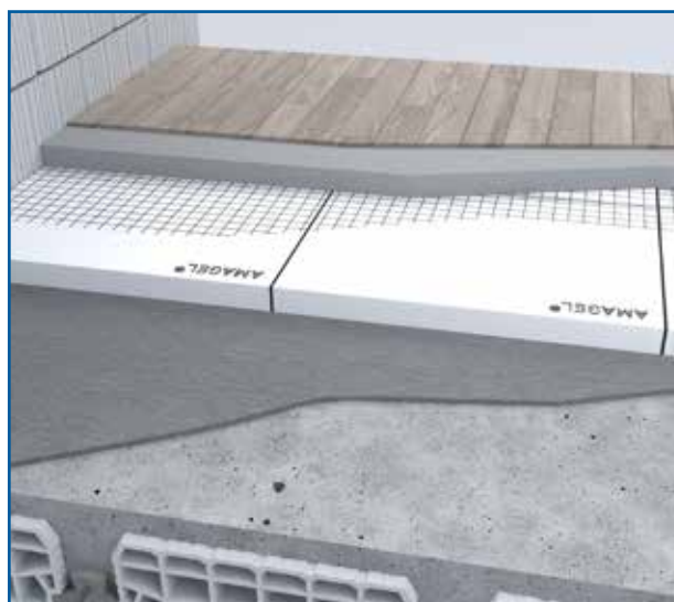
PLANCHERS INTERMÉDIAIRES
