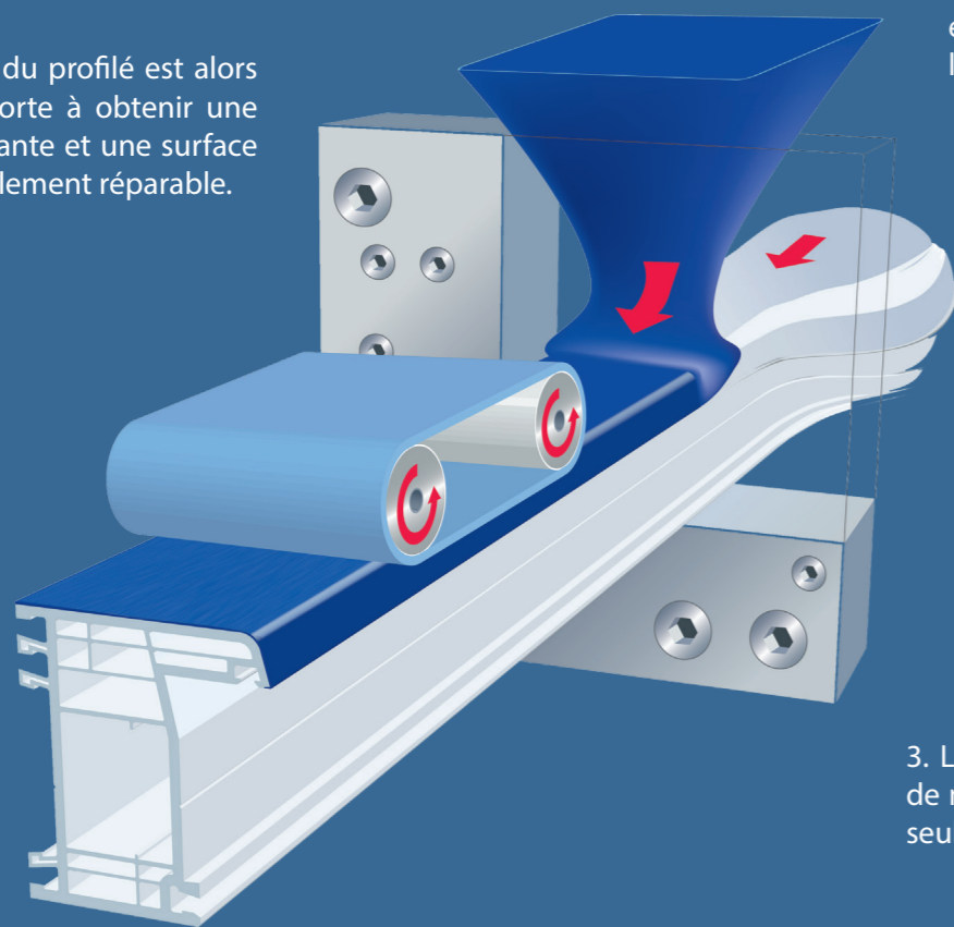
Profilé GEALAN-acrylcolor®
