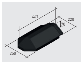
Q122*K | Remate cumbreira angular klinker
