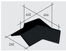
Q111*K | Cumbre ática 120° a 3 aguas klinker
