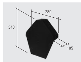
Q147*K | Tapón 45° klinker
