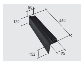
Q115*K | Remate lateral izquierdo Innova/Vienna klinker
