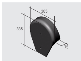
Q83*K | Tapón cumbreira circular klinker
