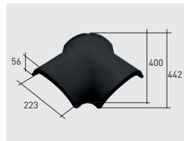
Q55*K | Cumbre redonda a 3 aguas klinker
