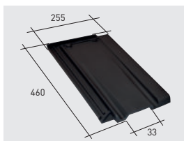
Q117*K | Teja ventilación Innova/Vienna klinker
