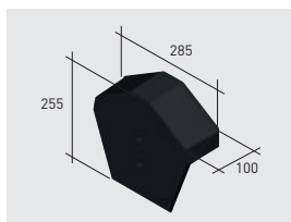
Q124*K | Tapón cumbreira angular klinker
