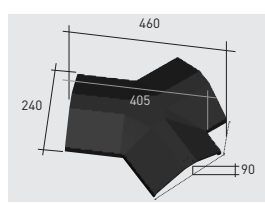
Q123*K | Cumbre angular a 3 aguas klinker
