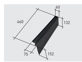
Q116*K | Remate lateral derecho Innova/Vienna klinker
