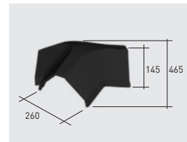
Q146*K | Cumbre pirámide a 3 aguas klinker
