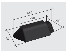
Q109*K | Remate cumbreira ática 120° klinker
