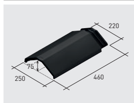
Q120*K | Cumbreira angular klinker
