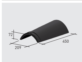
Q02*K | Cumbreira circular klinker
