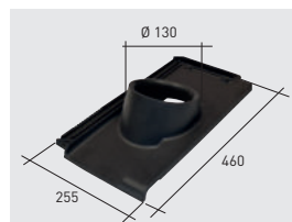
Q118*K | Teja soporte chimenea Innova/Vienna klinker
