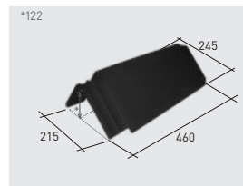
Q145*K | Cumbreira 45° klinker
