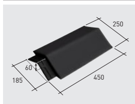
Q90*K | Cumbreira ática 120° klinker
