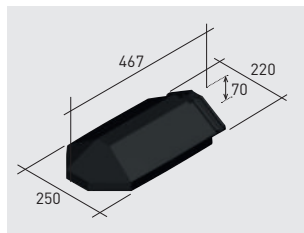
Q122*K | Remate cumbreira angular klinker
