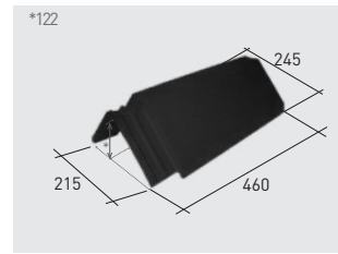
Q145*K | Cumbreira 45° klinker
