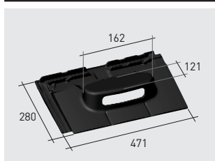
Q97*K | Visum3 chimenea klinker CAM87 | Visum3 rejilla chimenea klinker
