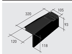
● Q99*K | Remate lat. derecho Visum3 klinker ● Q107*K | Remate lat. der. alero Visum3 klinker
