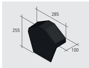
Q124*K | Tapón cumbreira angular klinker
