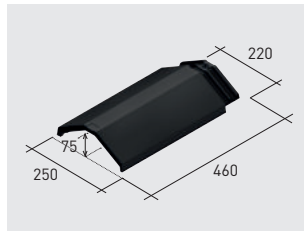
Q120*K | Cumbreira angular klinker
