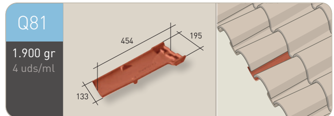
Alero canal igual pendiente
