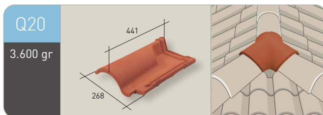
Teja de ventilación mixta pequeña
