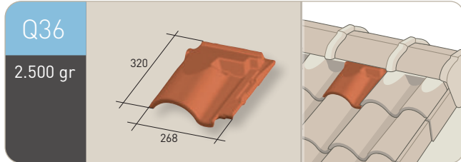
Alero cobija igual pendiente
