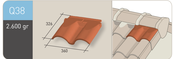
Alero canal igual pendiente
