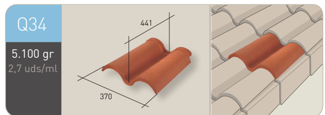
Doble teja mixta pequeña
