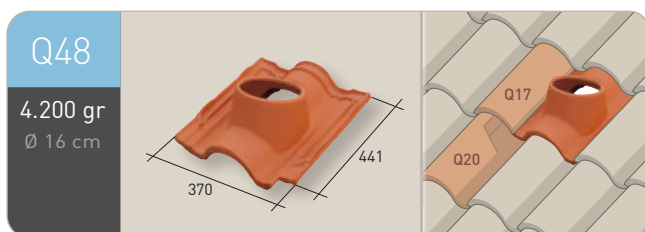
Teja soporte chimenea mixta pequeña (kit chimenea 160 mm)
