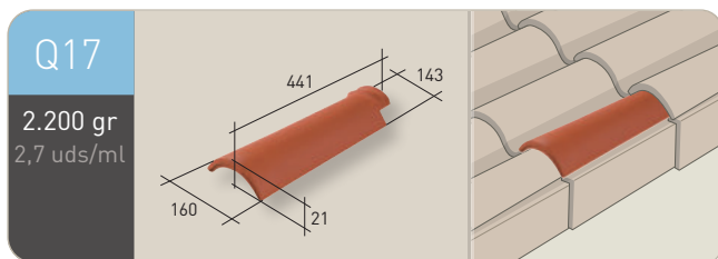
Media teja mixta pequeña
