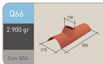
Soporte chimenea curva 50
