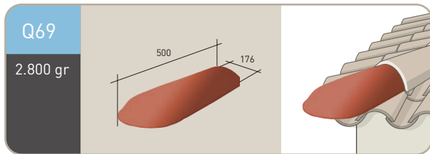
Tapón cumbrera circular
