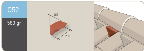
Remate lateral curvo izquierdo
