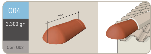
Tapón curva 50
