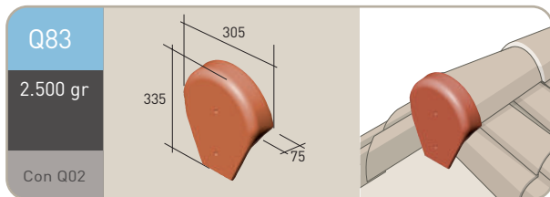
Cuña teja curva 40x15
