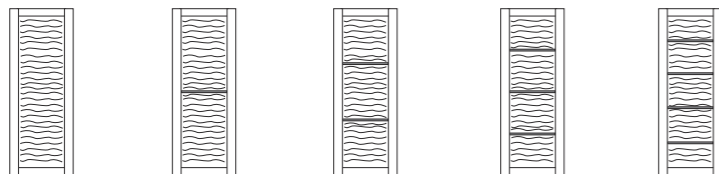
cieca blank Cieca con 1 inserto in acciaio Blank with 1 steel insert Cieca con 2 inserti in acciaio Blank with 2 steel inserts Cieca con 3 inserti in acciaio Blank with 3 steel inserts Cieca con 4 inserti in acciaio Blank with 4 steel inserts
