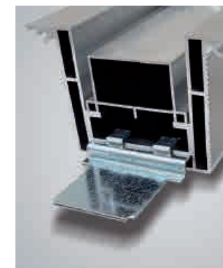
Montante di battuta in alluminio Aluminum stile
