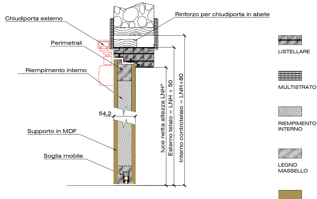
SEZIONE LONGITUDINALE
