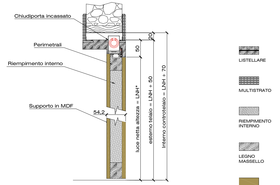
SEZIONE LONGITUDINALE
