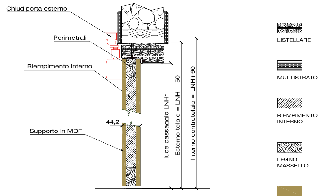
SEZIONE LONGITUDINALE
