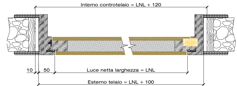
SEZIONE TRASVERSALE
