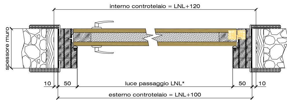
SEZIONE TRASVERSALE
