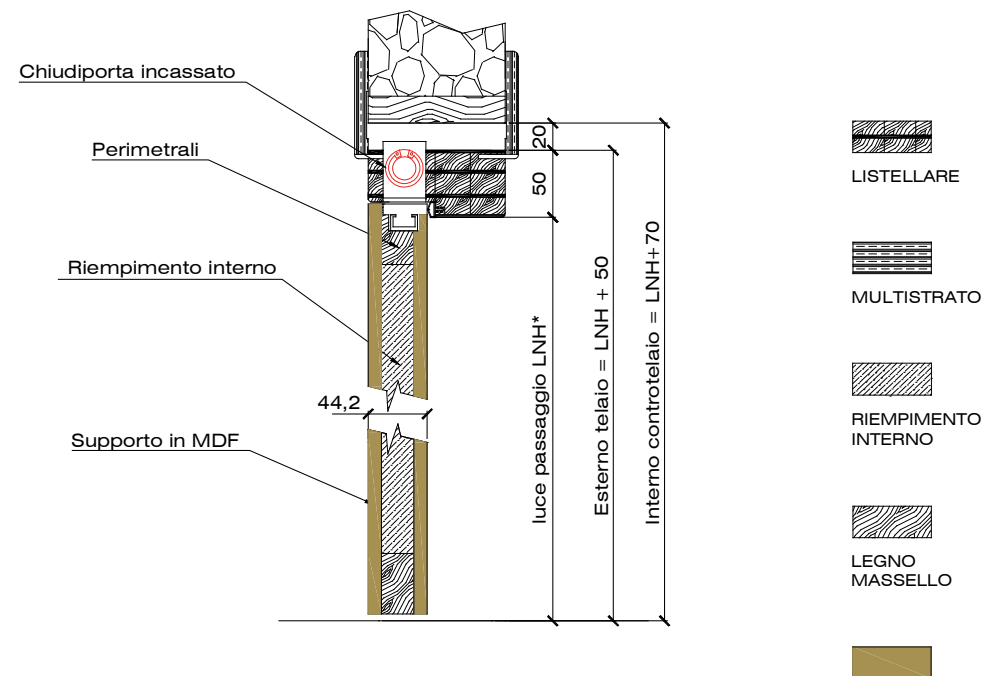
SEZIONE LONGITUDINALE
