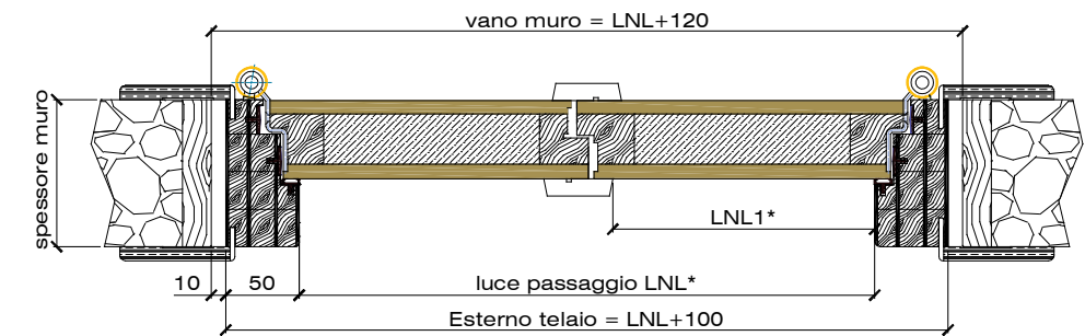
SEZIONE TRASVERSALE
