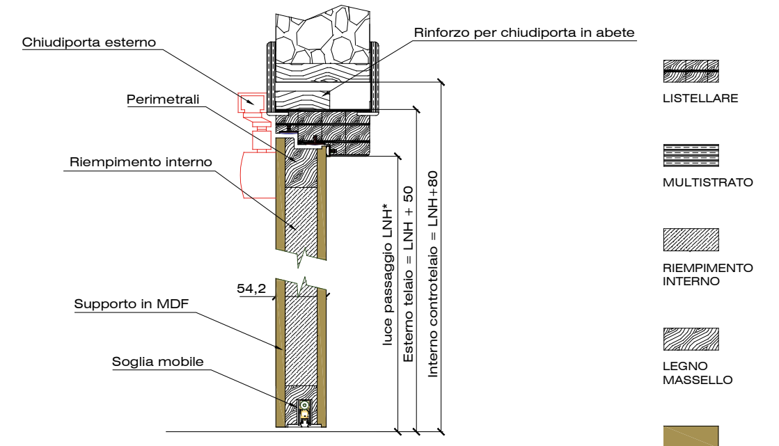
SEZIONE LONGITUDINALE
