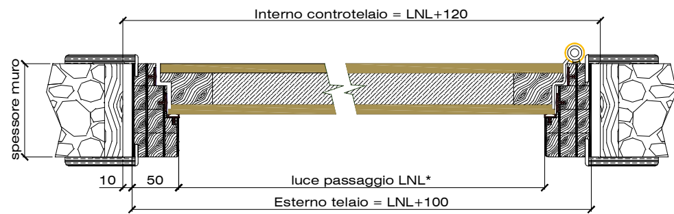
SEZIONE TRASVERSALE
