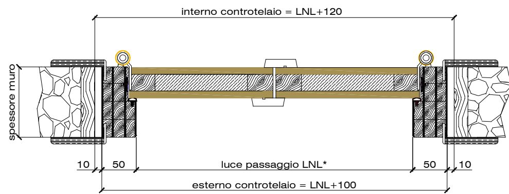
SEZIONE TRASVERSALE
