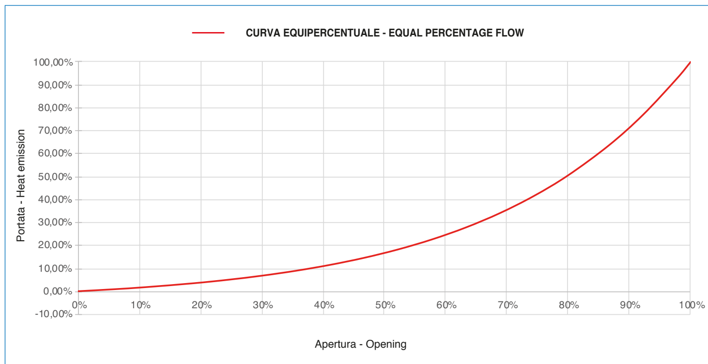
CURVA EQUIPERCENTUALE TIPICA DI VALVOLA DI REGOLAZIONE EQUAL PERCENTAGE FLOW TYPICAL OF CHARACTERIZED CONTROL VALVE
