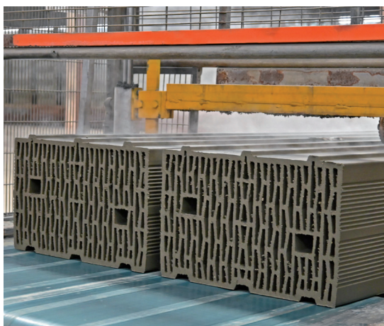
L'estrusione del prodotto "verde" dalla mattoniera
