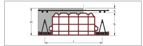
Solaio monotrave
