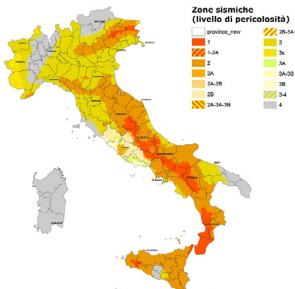
Mappa classificazione sismica del territorio italiano
