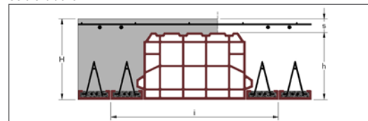
Solaio bitrave
