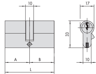
ARTÍCULO ON3S1, OA3S1, OP3S1
