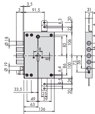
SERIE B6515, B7515, B7665
