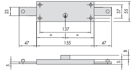
S B 1.41210.78 20 6,5 1.41320.78 17 9,5 1.41410.78 15 6 1.41510.78 15 5,5
