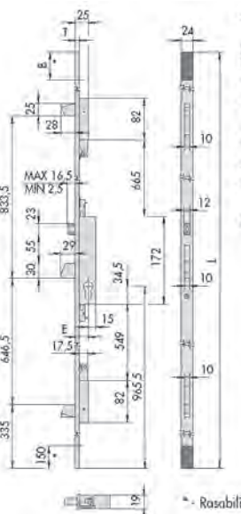
SERIE L T B 46450 2600 7 650 46650 2300 7 350 46550 2600 3 650 46750 2300 3 350 E = 25 - 30 - 35
