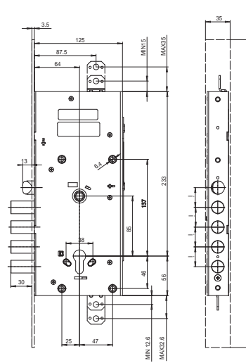
ARTÍCULO E6516, E6517, E6536, E6537
