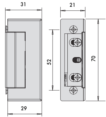
ARTÍCULO 15100, 15101, 15110, 15120, 15121, 15130, 15140, 15150
