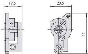
SERIE O2400
