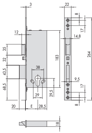
SERIE 12010, 12011 E = 40 - 50 - 60 - 70
