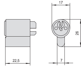
ARTÍCULO ON610, OQ610, OA610, OM610, OP610, OR610
