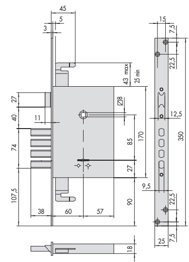
SERIE 57265
