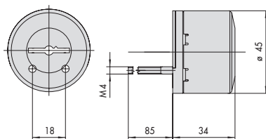
SERIE 02715, 02716
