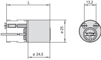
ARTÍCULO OG200, ON210, OQ210, OA210, OM210, OP210, OR210
