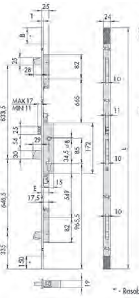
SERIE L T B 46425 2600 7 650 46625 2300 7 350 46600 1920 7 150 46525 2600 3 650 46725 2300 3 350 46700 1920 3 150 E = 25 - 30 - 35
