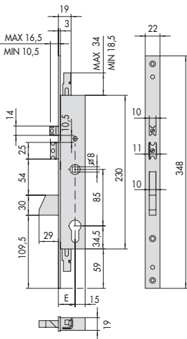
SERIE 16225 E = 25 - 30 - 35
