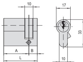
ARTÍCULO 0B030, 0G304, 0E304, 0Q314, 0N314, 0N324, 0A314, 0M324, 0P314
