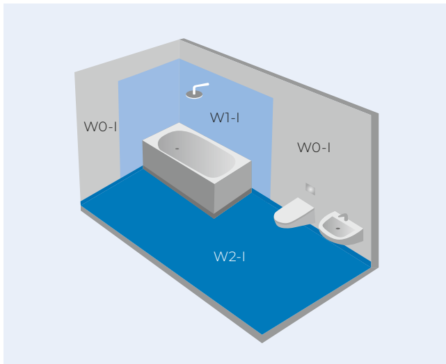
Abb. 1 Häusliches Bad mit Badewanne mit Brause ohne Duschartrennung
