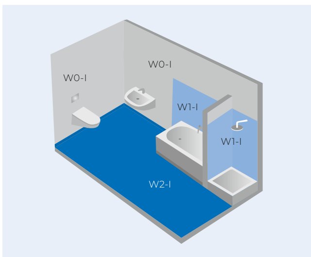
Abb. 2 Häusliches Bad mit Badewanne (ggf. mit Handbrause) und mit Duschtasse ohne Duschartrennung
