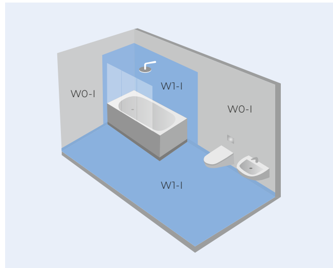
Abb. 3 Häusliches Bad mit Badewanne mit Brause und Duschartrennung
