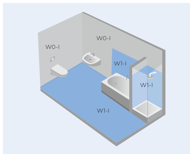
Abb. 4 Häusliches Bad mit Badewanne (ggf. mit Handbrause) und mit Duschtasse mit Duschartrennung
