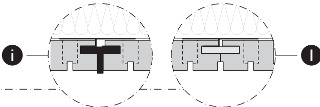
ANGOLO INTERNO A 90° 90° INTERNAL CORNER
