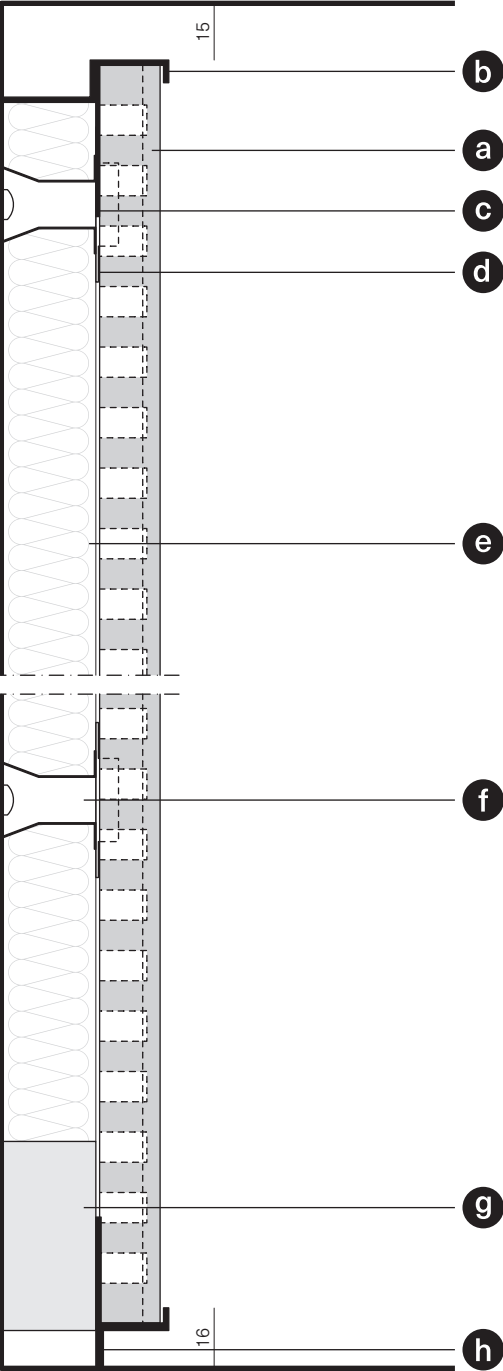
SEZIONE VERTICALE VERTICAL SECTION
