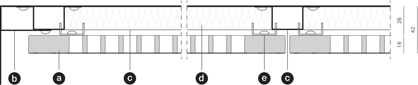
SEZIONE ORIZZONTALE HORIZONTAL SECTION
