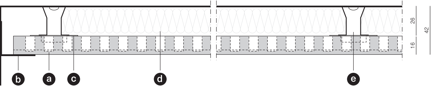
SEZIONE "TIPO" LONGITUDINALE TYPICAL LONGITUDINAL SECTION
