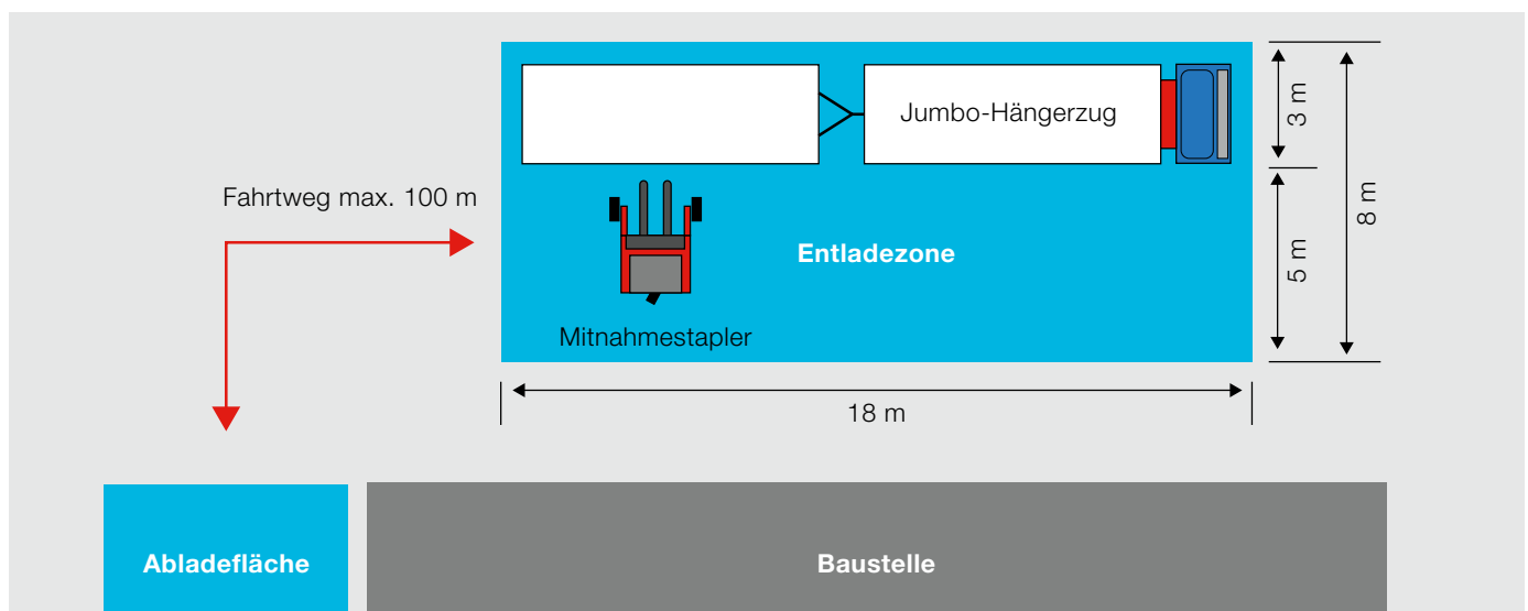
Mitnahmestapler: Eigengewicht: ca. 2 t Breite: ca. 2,3 m Masthöhe: ca. 2,4 m
