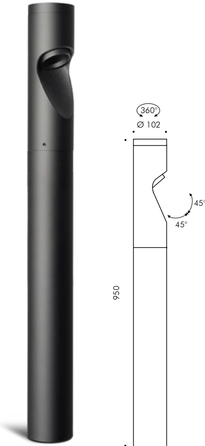
SHIFT POLLER H 950mm 1 Kopf
