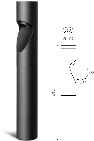
SHIFT POLLER H 635mm 1 Kopf
