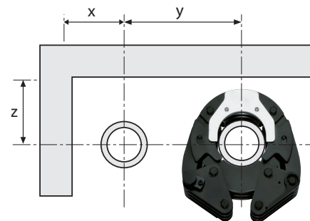
Fig. 52 - Distancias mínimas para mordaza de cadena 42-108.
