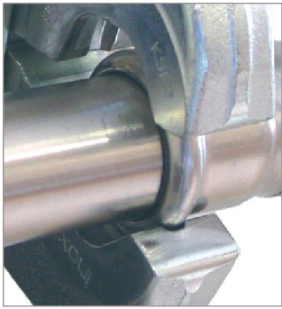
Fig. 55 - Introducir la ranura de la mordaza en el resalte del accesorio.
