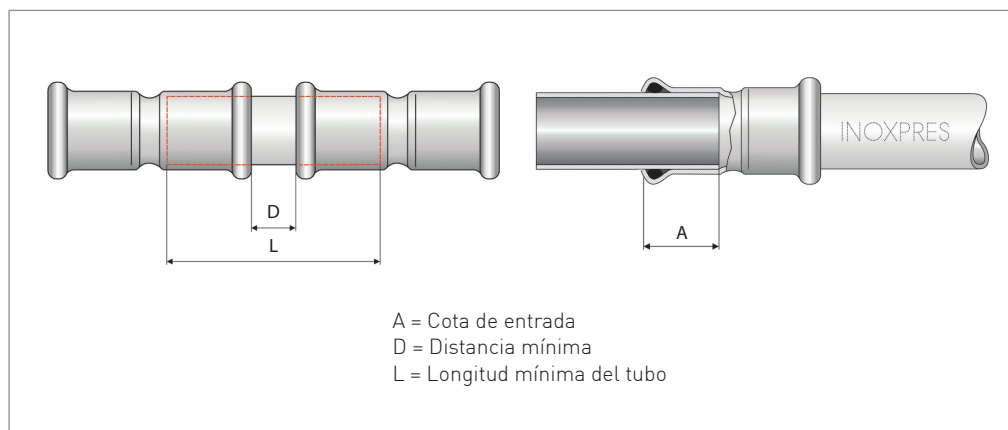
Fig. 47 - Distancias mínimas de montaje.
