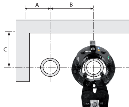
Fig. 53 - Distancias mínimas para mordaza de cadena 139,7-169,3.
