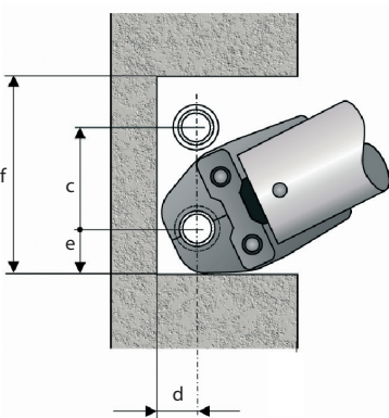
Fig. 50 - Distancias mínimas para mordazas de pinza 15-35 mm.
