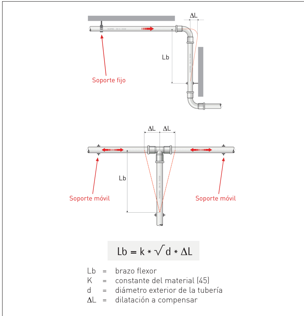
Fig. 63a - Cálculo brazo dilatación para posición ortogonal y T (ver tabla 26).
