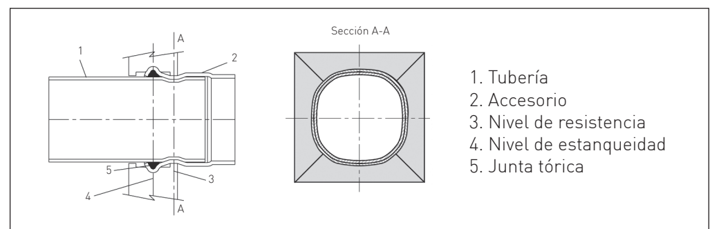
Fig. 2c - Vista en sección de la unión inoxPRES® para diámetros entre 42 y 108 mm. La sección A-A obtenida corresponde a la mordaza fabricada por Klauke.
