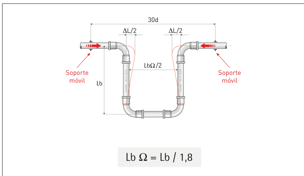
Fig. 63b - Cálculo brazo dilatación para posición en U (ver tabla 26).
