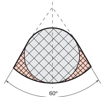
Fig. 32 - Junta INOXPRES
