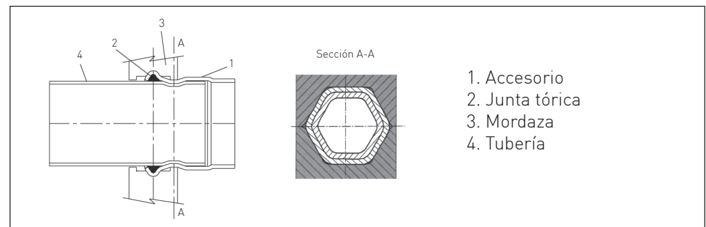
Fig. 2b - Vista en sección de la unión inoxPRES® para diámetros entre 15 y 35 mm. Se obtiene una sección hexagonal.
