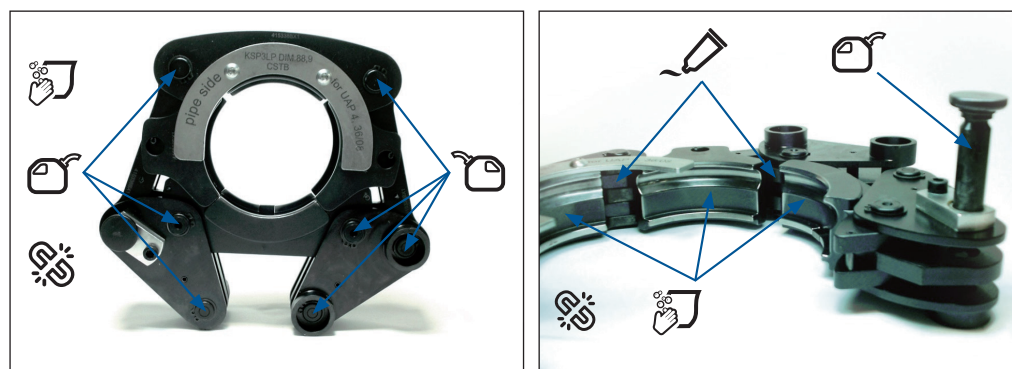
Fig. 58b - Mordaza Klauke UAP 100120 CFM bien introducida PENSAR.
