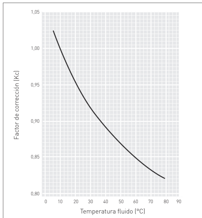
Fig. 65 - Para diferentes temperaturas de agua podemos utilizar el nomograma que en función de la temperatura del fluido indica el factor de corrección [Kc].
