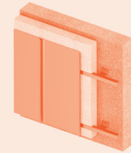
Sistema aislado sobre pared de hormigón
