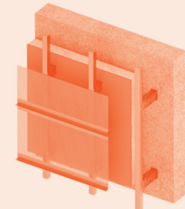
Sistema aislado sobre pared de hormigón con panel decorativo perforado
