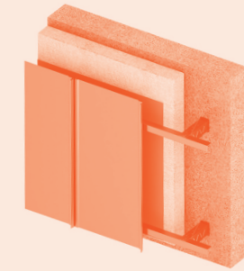
Sistema aislado ventilado sobre pared de hormigón
