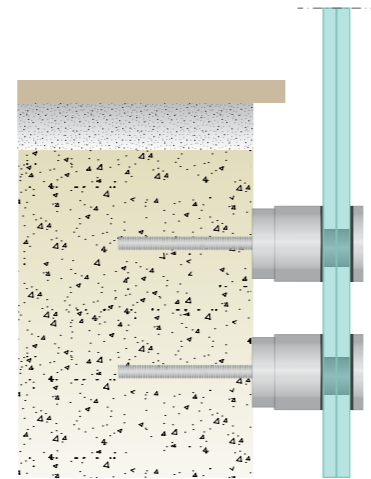
2 WITH OVERHANG/ AVEC REBORD External fixing/ Fixation extérieure
