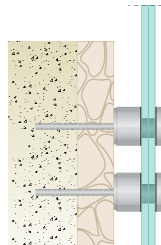
6 ON A STONE WALL SUR UN MUR EN PIERRE External fixing/ Fixation extérieure
