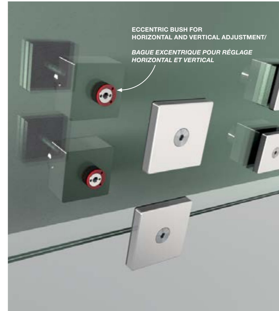
Exploded view of the accessory with detail of the eccentric bushing/ Vue éclatée de l'accessoire avec détail de la bague excentrique.
