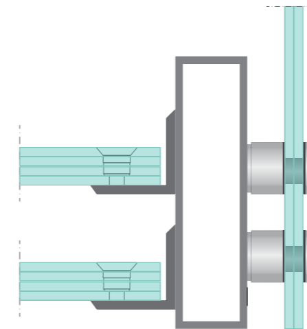
3 ON A STAIRCASE SUR UN ESCALIER External fixing/ Fixation extérieure
