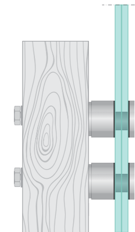
4 ON A WOODEN BEAM SUR UNE POUTRE EN BOIS External and internal fixing/ Fixation extérieure et intérieure
