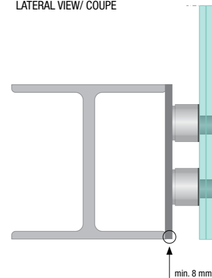
7 ON A DOUBLE T-BEAM SUR UNE POUTRE DOUBLE EN FORME DE T External and internal fixing/ Fixation extérieure et intérieure
