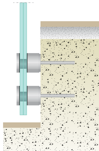
5 FROM THE INNER SIDE OF A LOW WALL À L'INTÉRIEUR D'UN MURET Internal fixing/ Fixation intérieure
