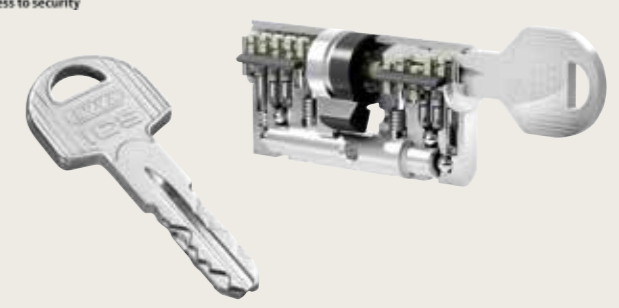
CILINDRO EUROPEO EVVA ICS AD ALTA SICUREZZA CYLINDRE EUROPÉEN EVVA ICS DE HAUTE SÉCURITÉ
