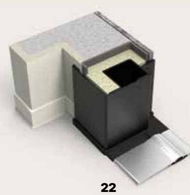
22 Controtelaio e telaio porta blindata a bilico Di.Big per rivestimento muro esterno. Subframe and frame for Di.Big pivot security door with exterior wall finish.
