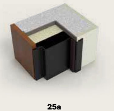
25a Controtelaio e telaio porta blindata RasoMuro per rivestimento muro interno. Subframe and frame for RasoMuro security door with interior wall finish.
