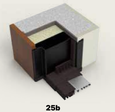
25b Controtelaio e telaio porta blindata RasoMuro per rivestimento muro interno e soglia a taglio termico e a barriera dell'acqua. Subframe and frame for RasoMuro security door with interior wall finish. Watertight threshold with thermal break.
