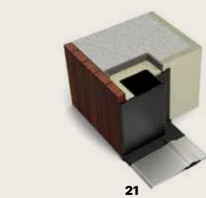
21 Controtelaio e telaio porta blindata a bilico Di.Big per rivestimento muro interno. Subframe and frame for Di.Big pivot security door with interior wall finish.
