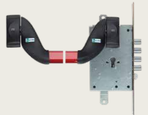
SERRATURA CON MANIGLIONE ANTI-PANICO LOCKING SYSTEM WITH PANIC EXIT DEVICE
