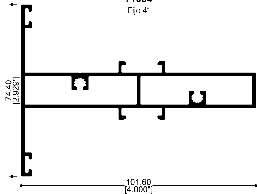
71251 Intermedio fijo
