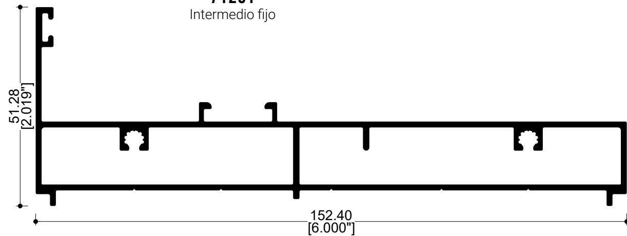
71253 Fijo 6"
