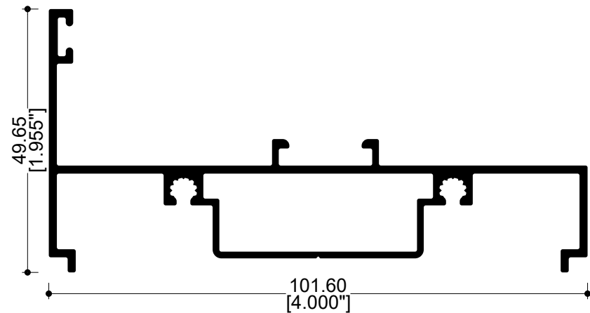
71354 Fijo 4"
