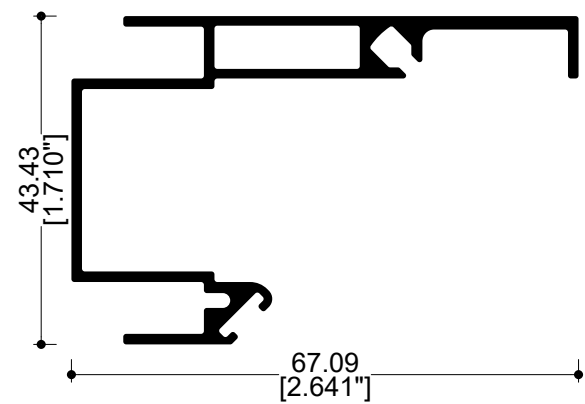
72536 Esquinero 90°
