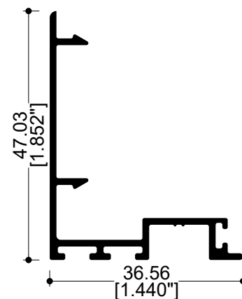
70952 Traslape 90°
