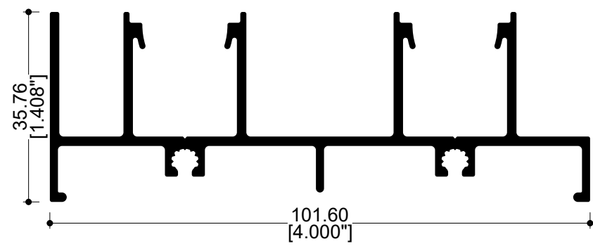
70942 Riel 2 pistas
