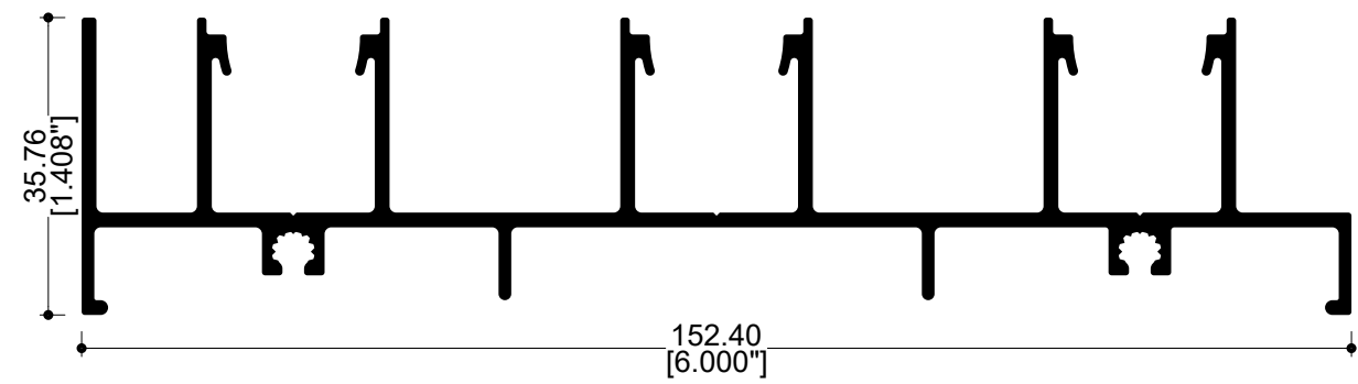
70943 Riel 3 pistas
