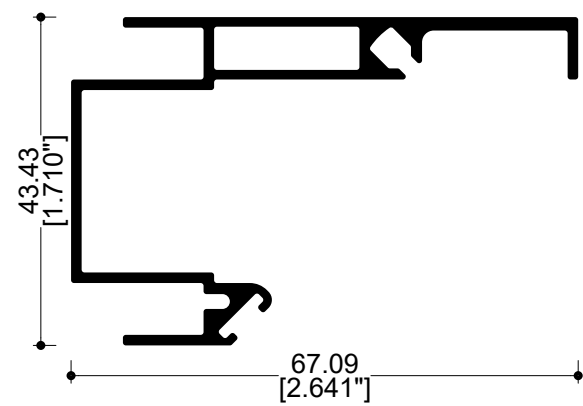
72536 Esquinero 90°
