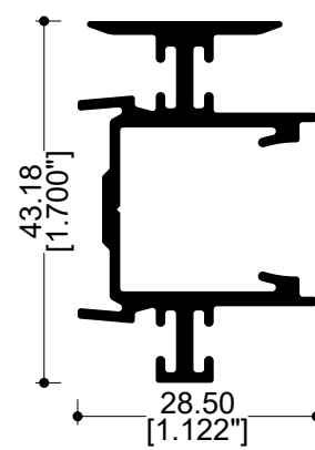
70956 Adaptador OXXO
