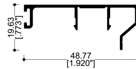
70954 Tapa vista
