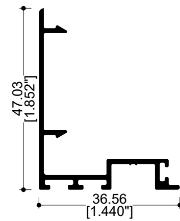
70952 Traslape 90°
