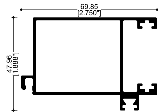
70950 Traslape mosquitero
