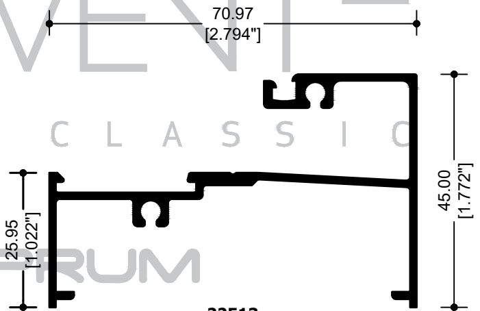
22513 ESCALONADO INTERIOR
