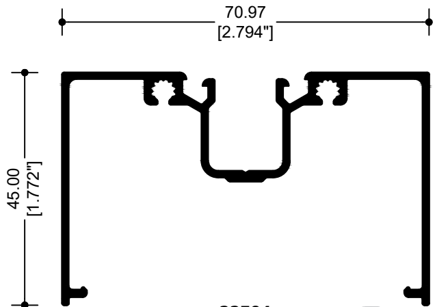
22504 BOLSA
