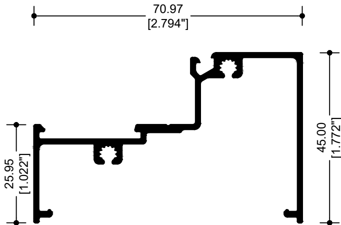
32506 ESCALONADO EXTERIOR
