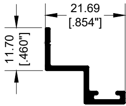
50701 ADAPTADOR OXO
