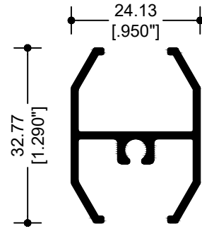
14918 PERFIL P/CUADRÍCULA
