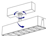
NATYNKOWA FLEX 340° 90° SURFACE MOUNTED FLEX 340° 90°
