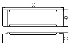
TRETO IP67 48V 100W
