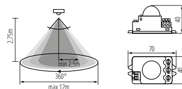
ROLF MINI IO-L
