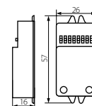
DABA AIO MW SENSOR
