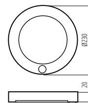
ERGA PIR 10-18W CCT
