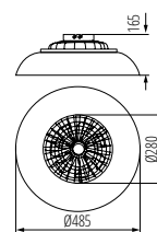
PLAVE PAN48 CCT+RGB W
