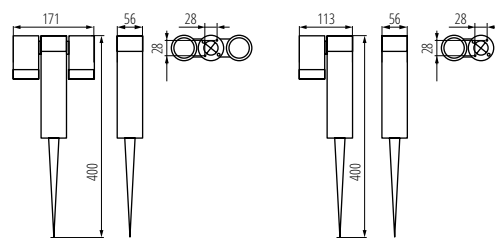
USTI SP 2X7 GR
