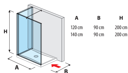
glass wall „L“ 120, 140 x 90 cm
