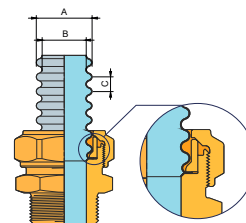
DIMENSIONI TUBO CONSIGLIATE
