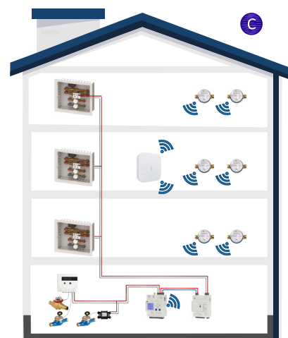
SISTEMA MISTO CABLATO + RADIO
