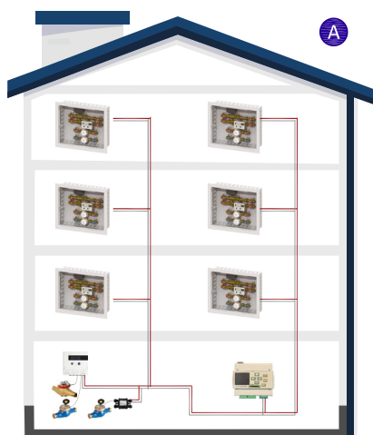
SISTEMA CABLATO ≤ 250 UNITÀ'
