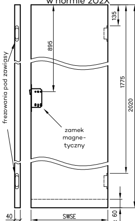
Skrzydła Sara Eco 2 bezprzylgowe w normie 202X
