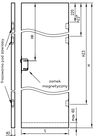
Skrzydła bezprzylgowe rozwiernie Standard 10, Modern, Plus
