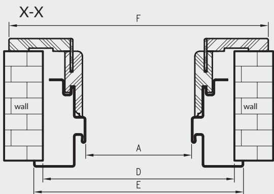
door frame profile
