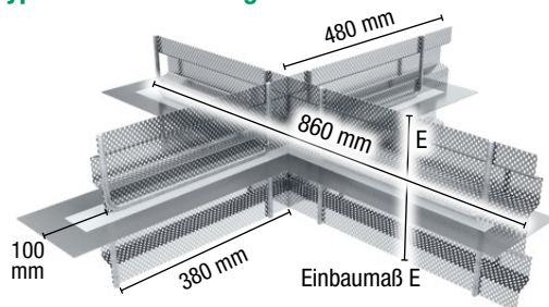
DICHTBLECH ABS Kreuz-Profil verzahnt – Typ S
