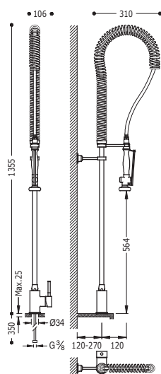
Bateria jednouchwytowa z wyciąganą wylewką do kuchni przemysłowej Z elastycznymi węzami zasilającymi G3/8.
